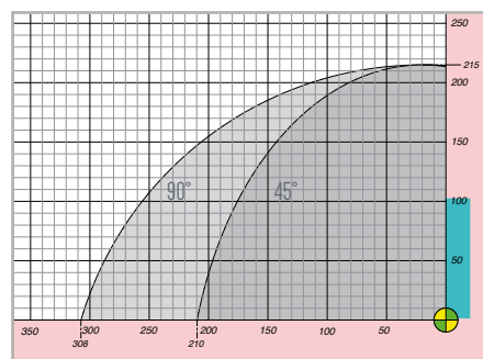
Diagramma di taglio / Cutting diagram Supporto del profilo in posizione standard / Profile support in the standard position
