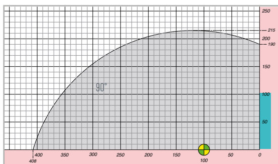
Diagramma di taglio / Cutting diagram Supporto del profilo in posizione arretrata / Profile support in the backward position
